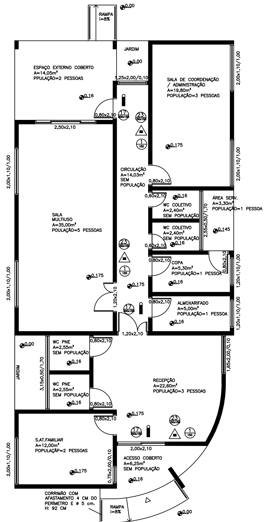
PLANTA BAIXA PPCI ÁREA: 165,30m 2 ESCALA 1:100
