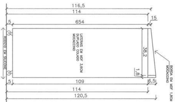
VISTA LATERAL DO PÚLPITO
